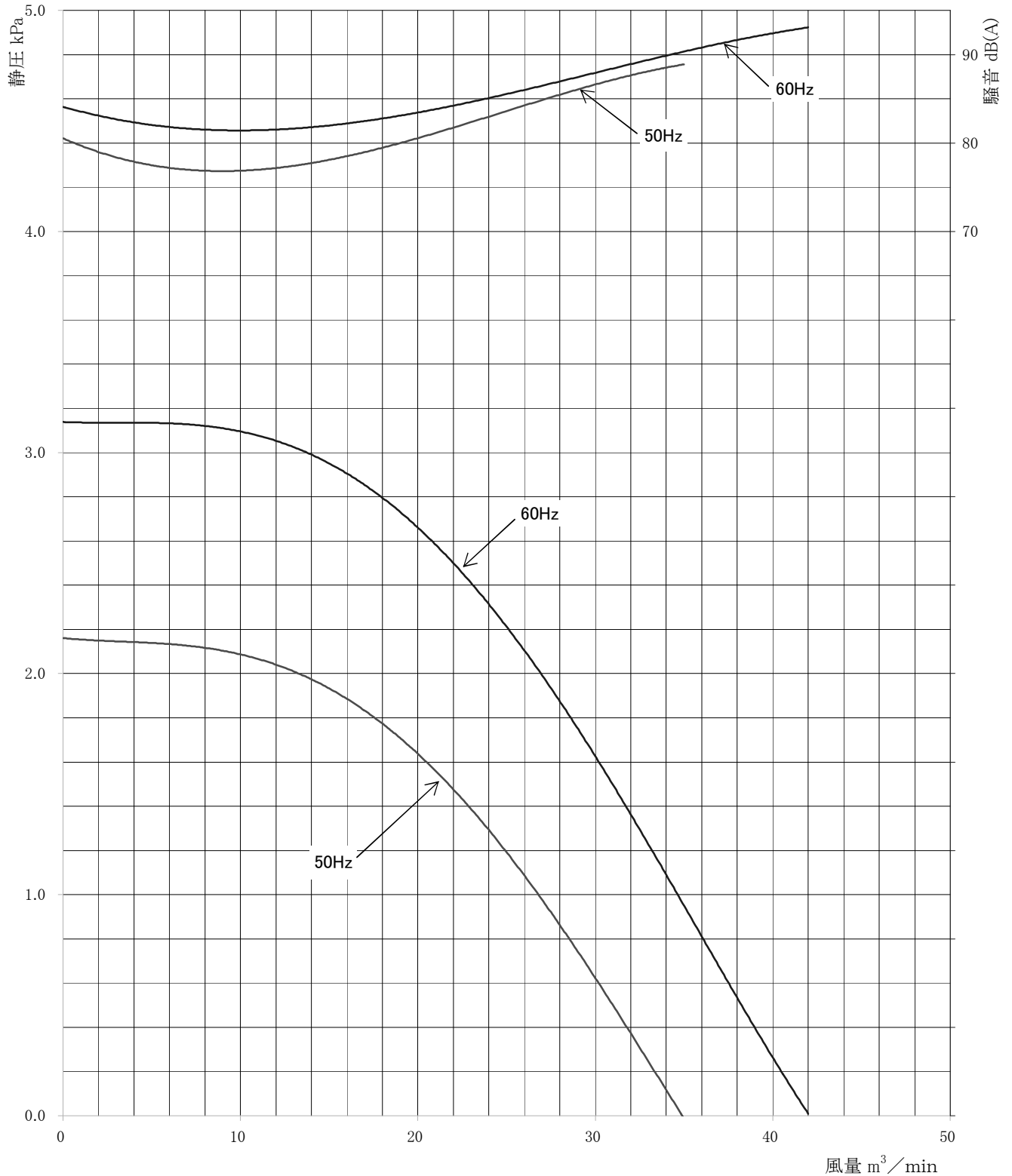
性 能 曲 線
