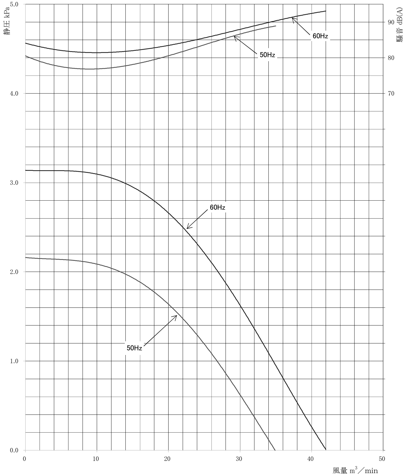
性 能 曲 線
