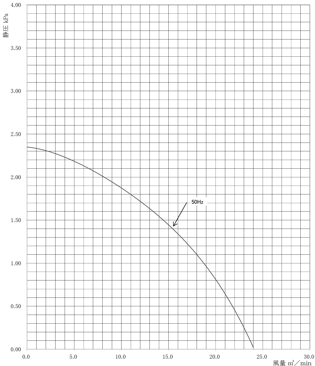
性 能 曲 線
