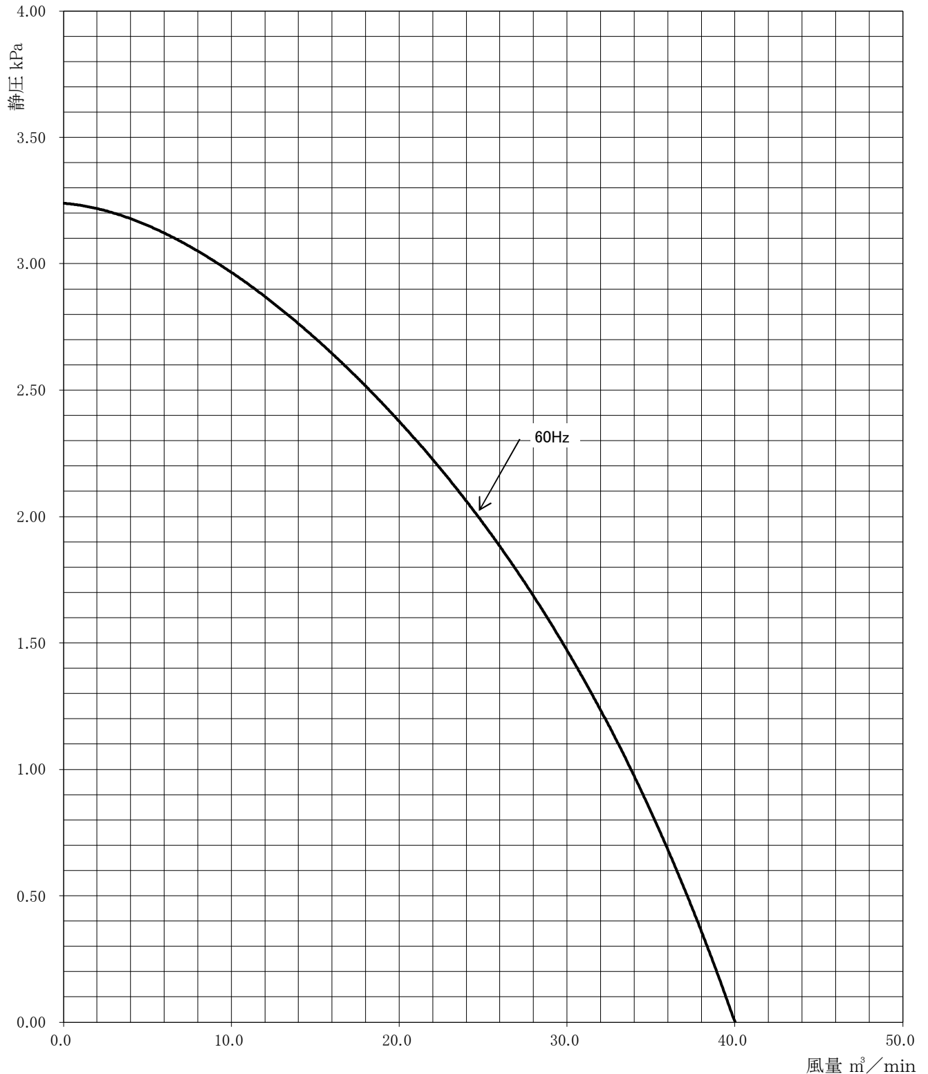
性 能 曲 線
