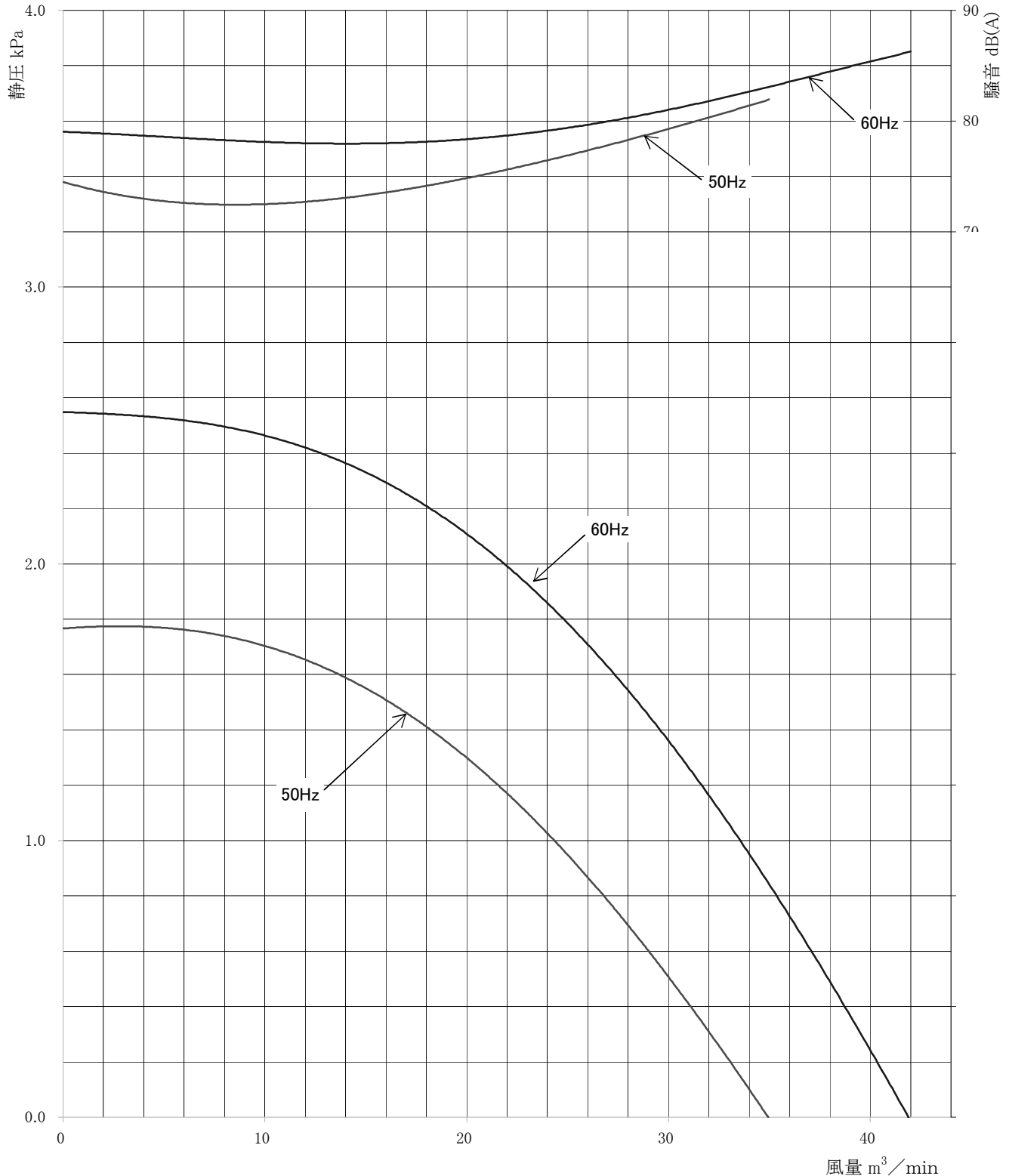
性 能 曲 線
