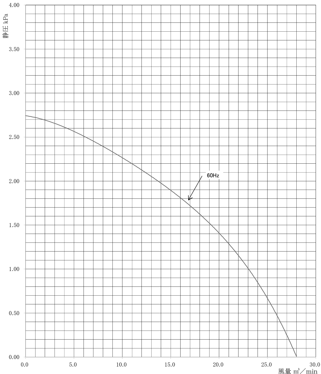
性 能 曲 線
