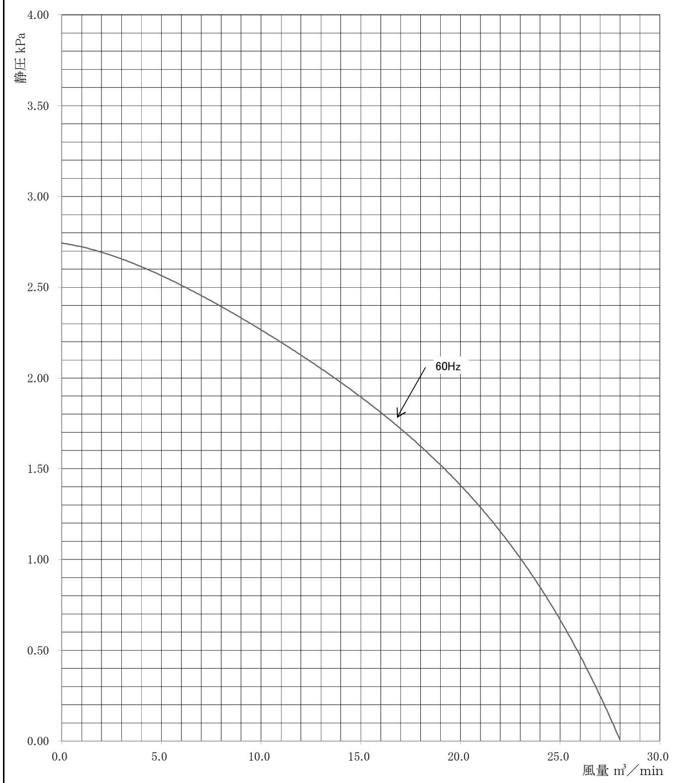
性 能 曲 線 20 °C 換 算 値
