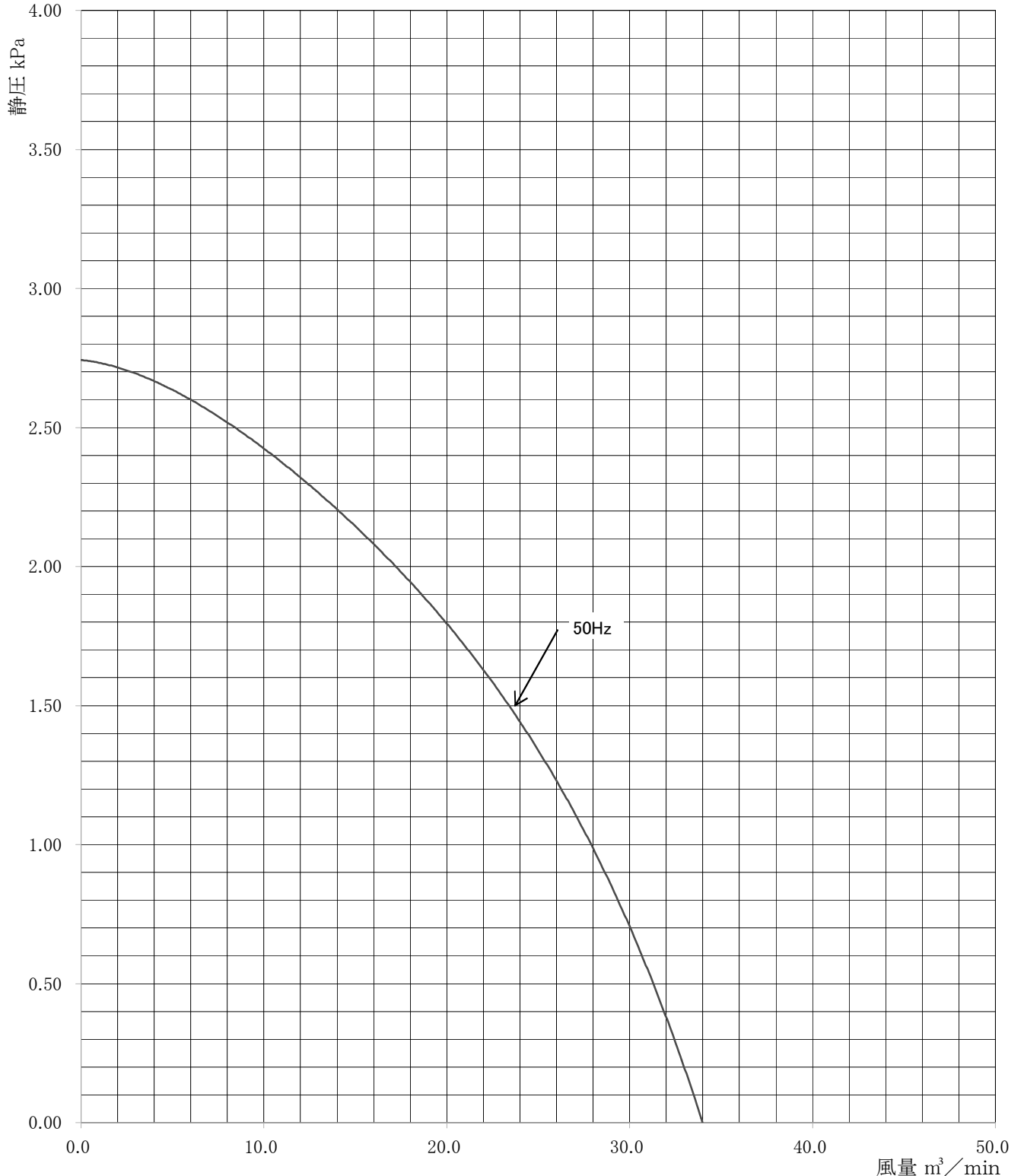
性 能 曲 線
