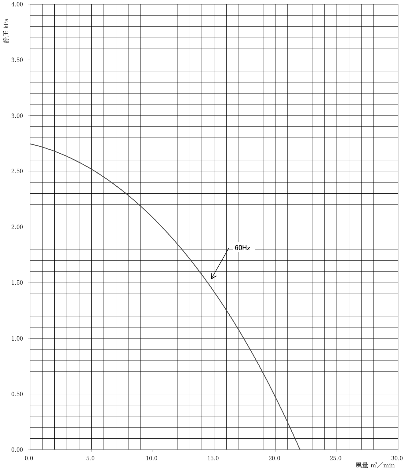
性 能 曲 線
