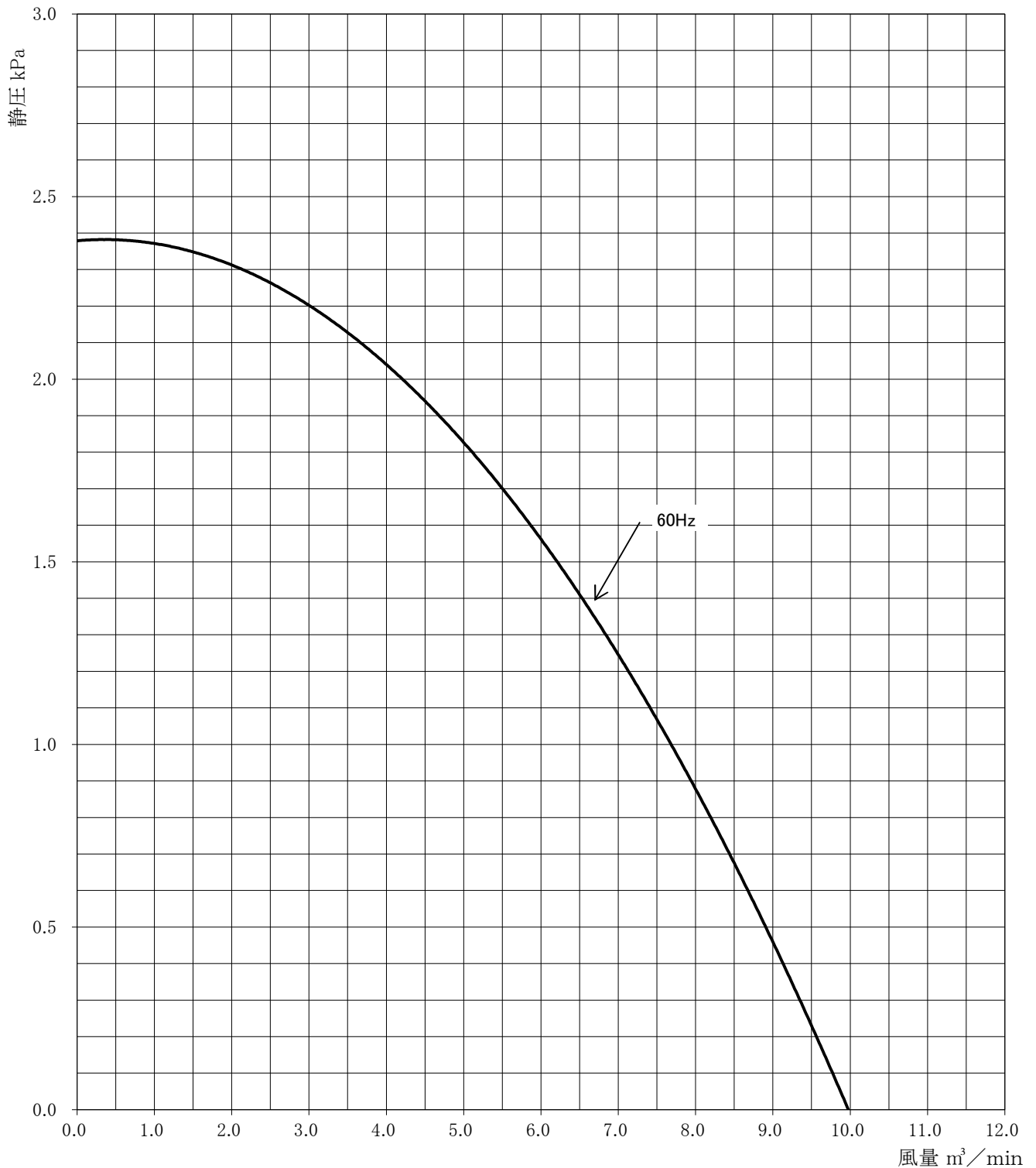
性 能 曲 線
