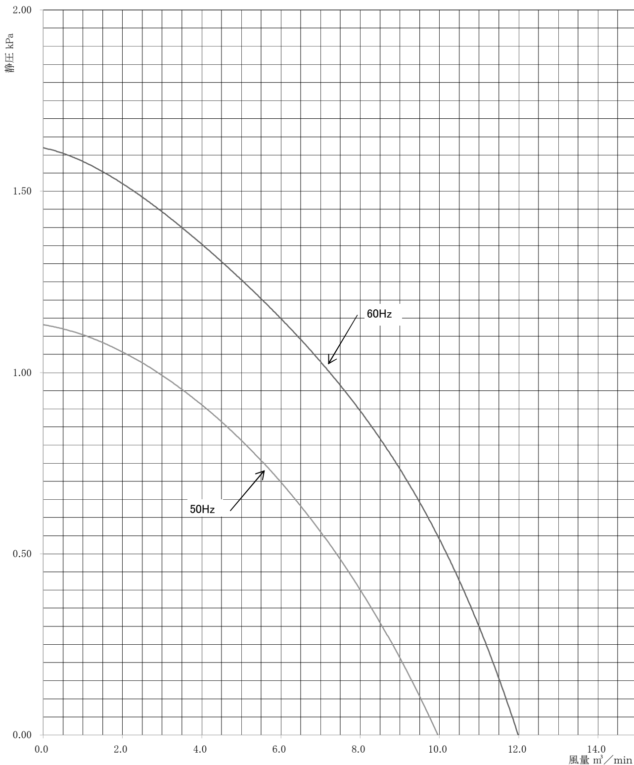
性 能 曲 線
