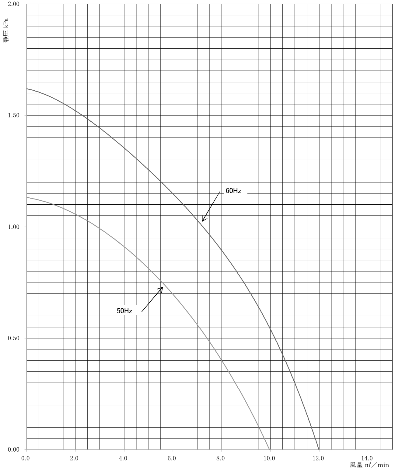
性 能 曲 線
