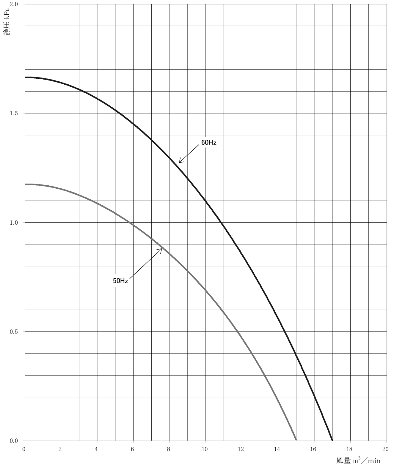
性 能 曲 線
