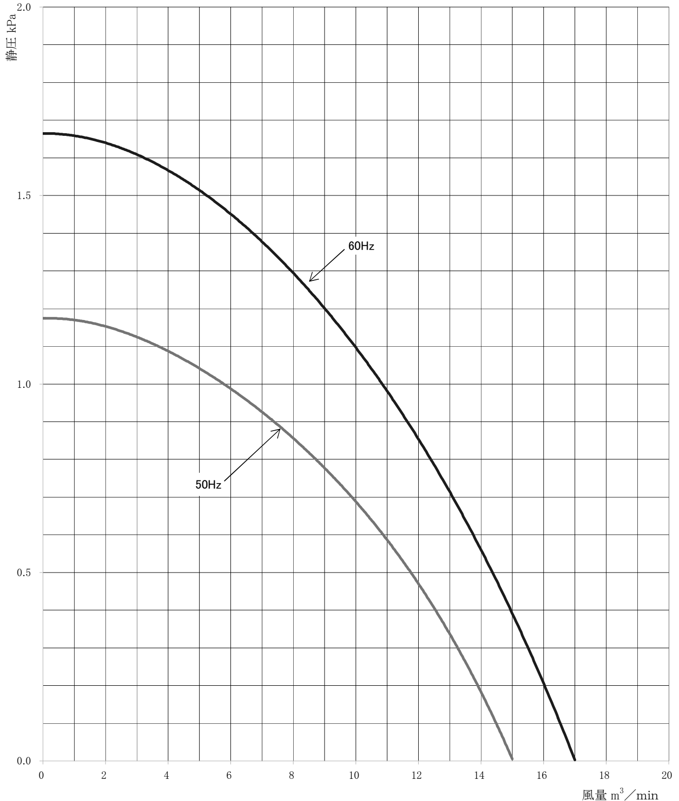
性 能 曲 線
