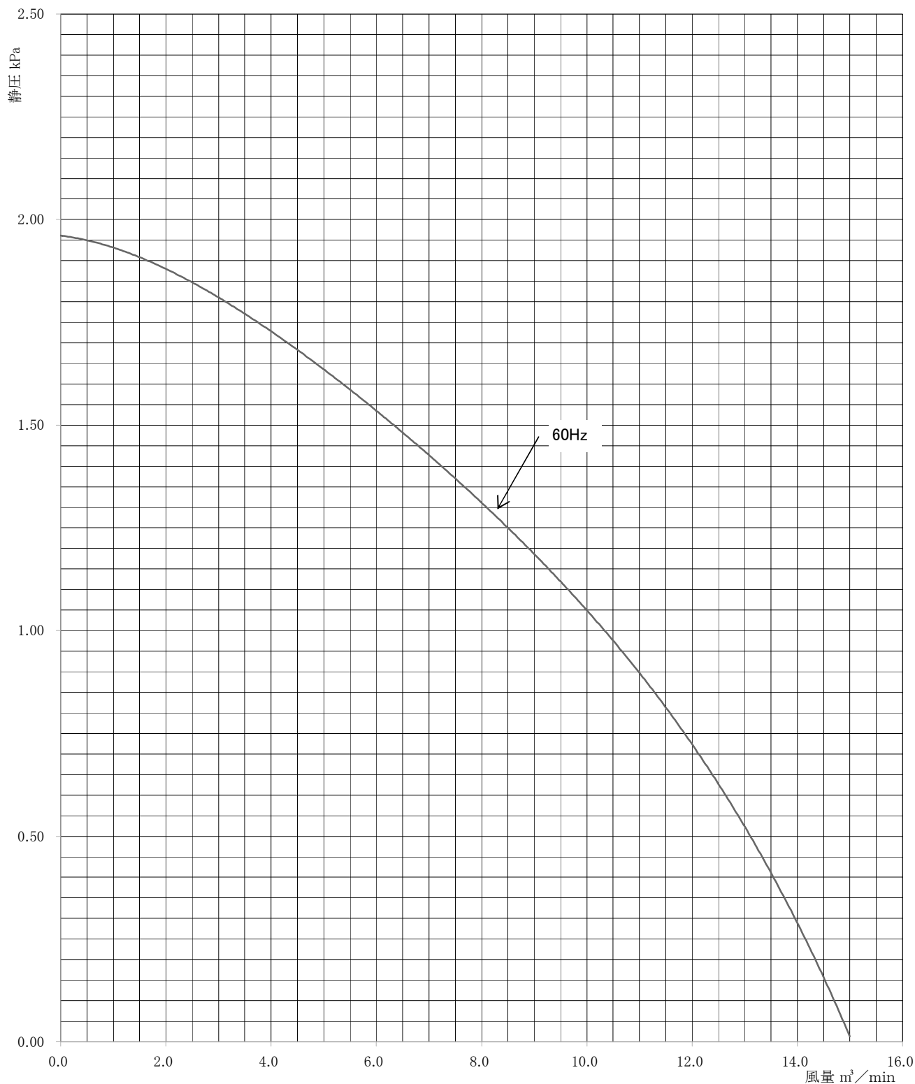
性 能 曲 線
